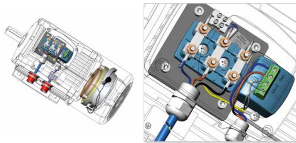
ATDC \Delta + conexión separada del rectificador 400Vac/180Vdc [fig. 4]
