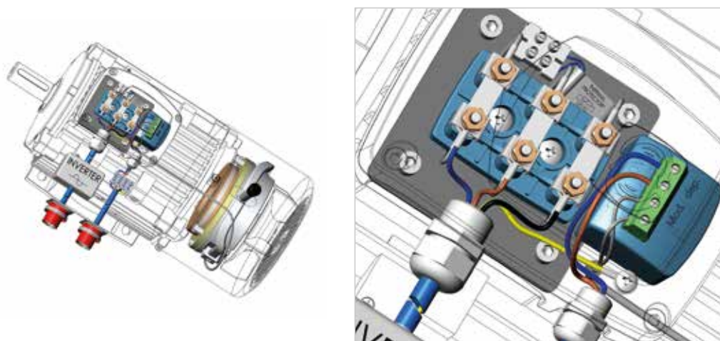
ATDC \Delta [conexión separada del rectificador 400Vac/180Vdc] + inverter [fig. 3]
